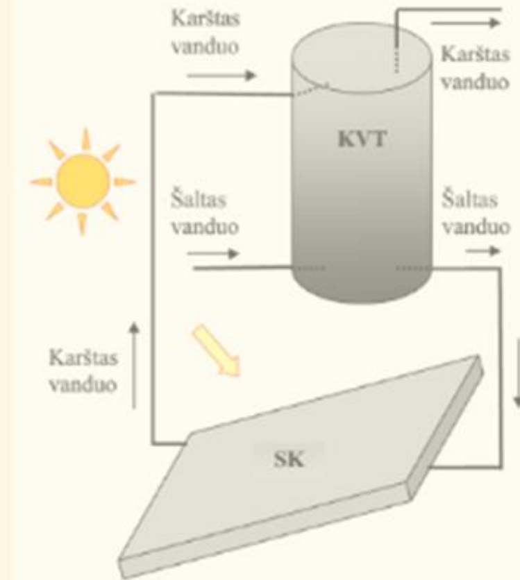
12 pav. Pasyvosios cirkuliacijos saulės kolektorių sistema [1 p.45]
